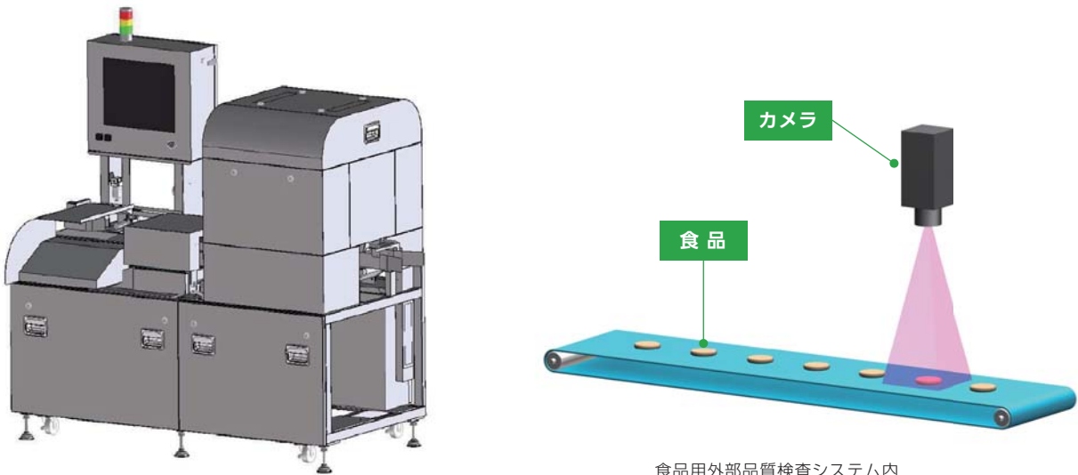
食品用外部品質検査システム外観
